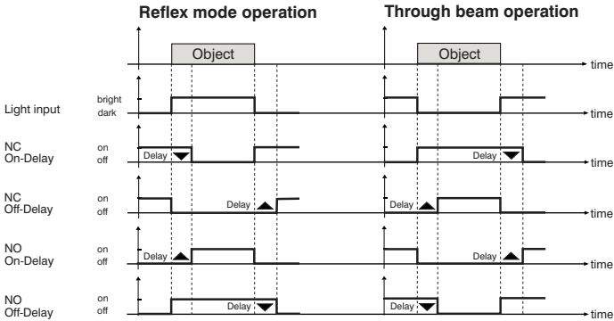
fig. 4 ON-/OFF-Delay
