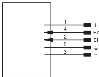
Emitter
