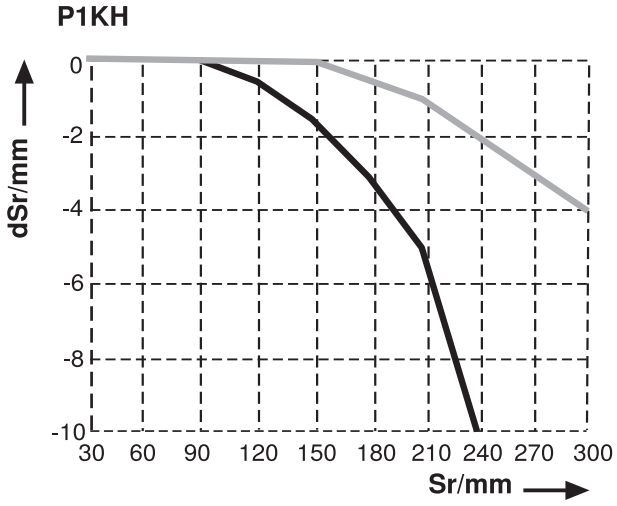
Şekil 1: Anahtarlama mesafesi sapması
