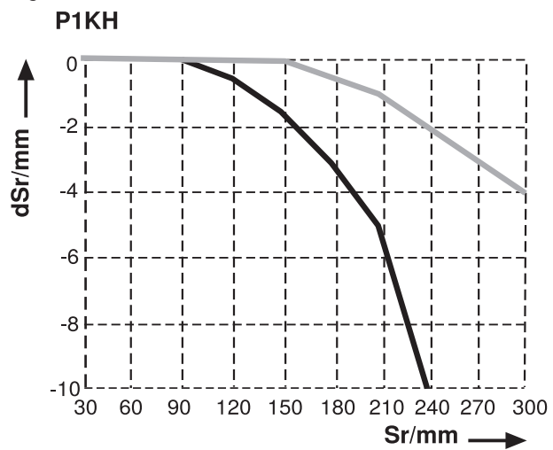
Fig. 1: Desviación distancia conmutación
