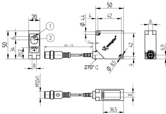
Maßangaben in mm / All dimensions in mm / Mesures en mm 1 = Sendediode / Transmitter diode / Diode émettrice 2 = Empfangsdiode / Receiver diode / Diode réceptrice Schraube / Screw / Vis M4 = 0,5 Nm
