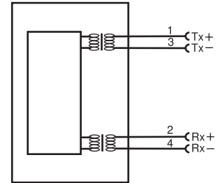
Ethernet bağlantı şeması
