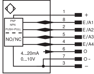
Besleme gerilimi bağlantı şeması
