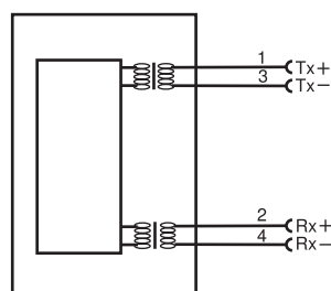
Esquema de conexión Ethernet
