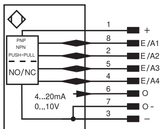
Esquema de conexión Tensión de alimentación
