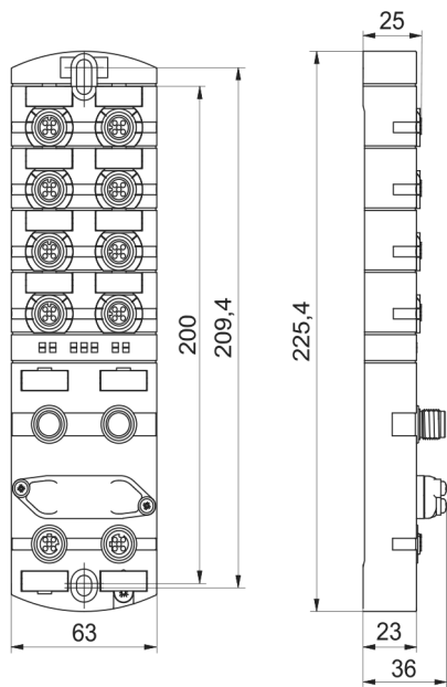
尺寸数据, 单位mm (1 mm = 0.03937 Inch)
