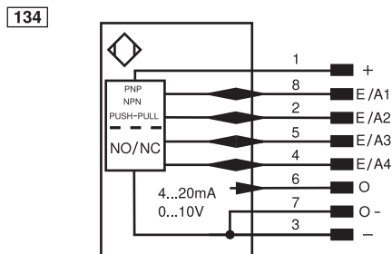
Anschlussbild Versorgungsspannung
