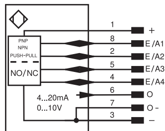
Anschlussbild Versorgungsspannung
