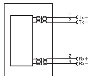
Anschlussbild Ethernet
