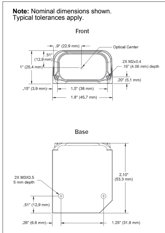
FIS-6300 Ultrascan Dimensions
