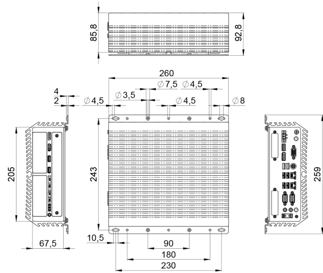
尺寸数据, 单位mm (1 mm = 0.03937 Inch)
