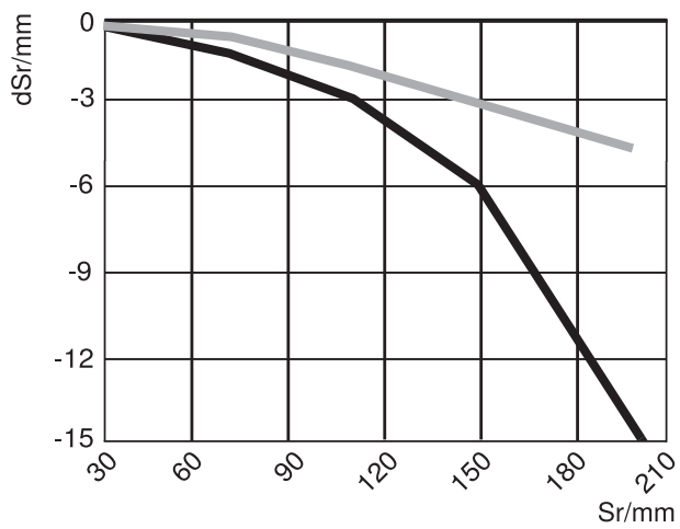
Abb. 1: Schaltabstandsabweichung
