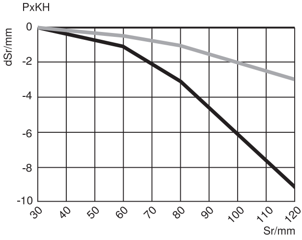
Şekil 1: Anahtarlama mesafesi sapması
