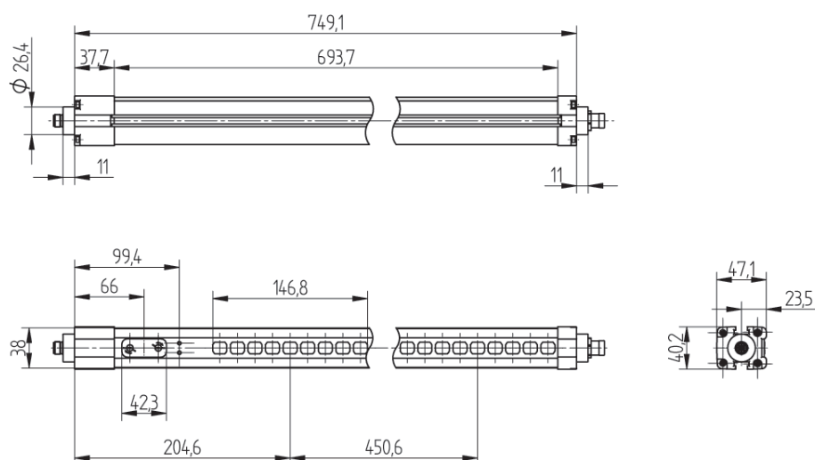
Emitter SB4-50IS050C1
