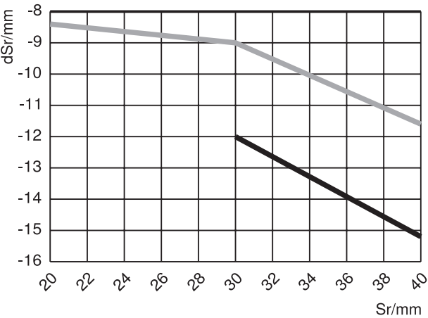
基于反射率90%的白色目标的典型特征曲线
