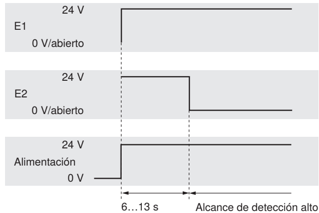
Diagrama de tiempo
