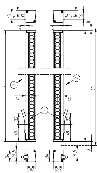
Maßangaben in mm / All dimensions in mm / Mesures en mm ① = Sender / Emitter / Emetteur ② = Empfänger / Receiver / Récepteur ③ = Bedienfeld / Ctrl. Panel / Panneau SFH = Schutzfeldhöhe / Protection Zone Height / Hauteur du champ de protection
