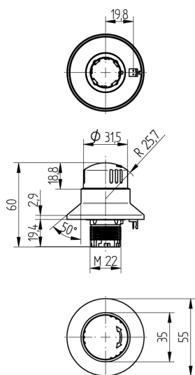
尺寸数据, 单位mm (1 mm = 0.03937 Inch)
