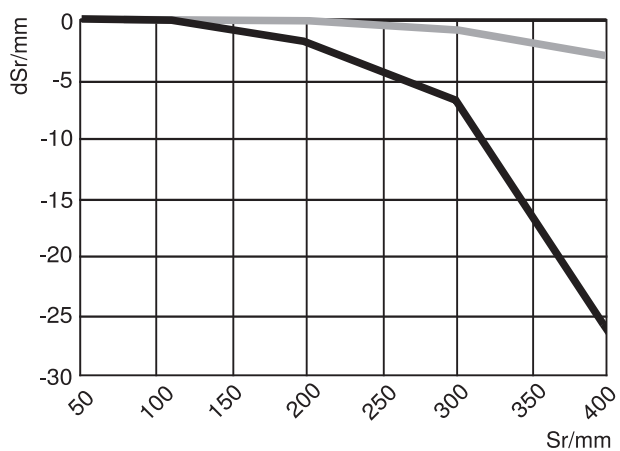
Fig. 1: Desviación distancia conmutación P1PH
