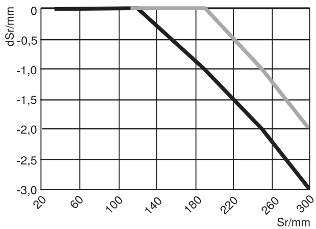
Fig. 1: Desviación distancia conmutación P1NH
