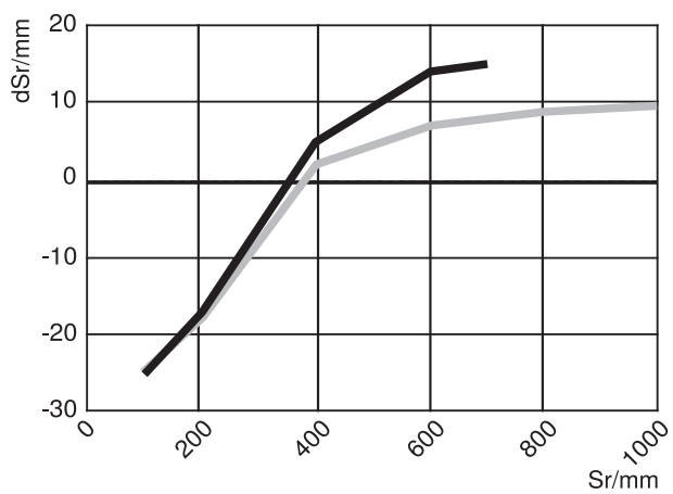
Fig. 1: Desviación distancia conmutación PxKY0
