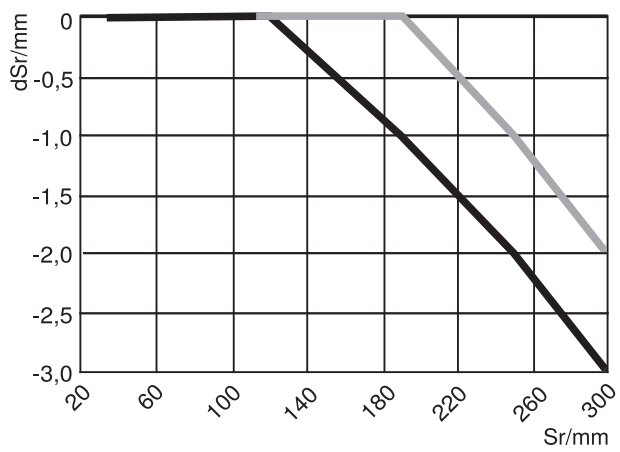
Abb. 1: Schaltabstandsabweichung
