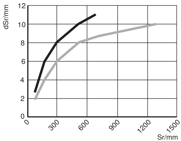
Abb. 1: Schaltabstandsabweichung P1KY1
