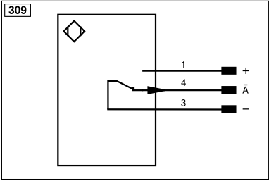
螺钉 M3 = 0,5 Nm 尺寸数据, 单位mm (1 mm = 0.03937 Inch)
