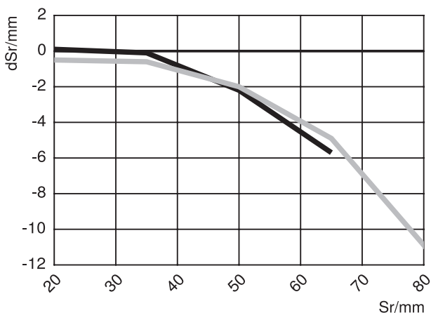
Fig. 1: Desviación distancia conmutación HO08
