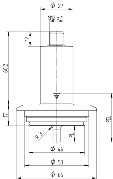
尺寸数据, 单位mm (1 mm = 0.03937 Inch)
